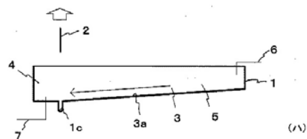
図1 植物用栽培装置の構造
